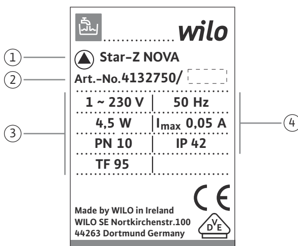
Kennzeichnung Typenschild Baureihe Wilo-Star-Z NOVA
