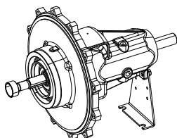
Рис. 18: Вставной блок
