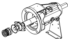
Рис. 22: Скользящее торцевое уплотнение
