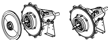
Рис. 17: Вставной блок
