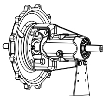
Рис. 19: Вставной блок
