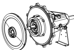
Рис. 37: Рабочее колесо
