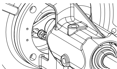
Рис. 32: Крышка скользящего торцевого уплотнения
