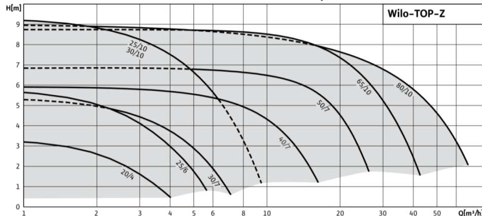
Štandardné 3-otáčkové cirkulačné čerpadlá:
