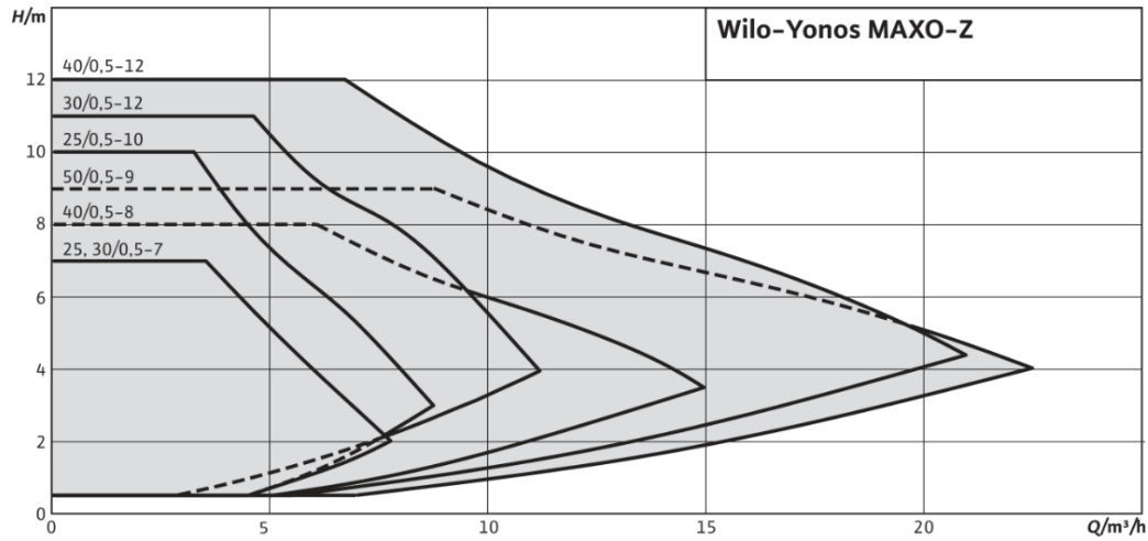
Štandardné úsporné cirkulačné čerpadlá TV
