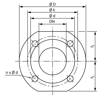
Flansch G
