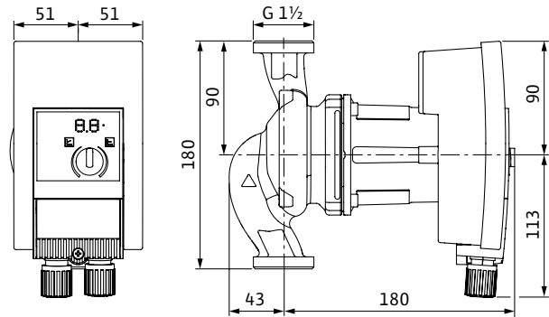
Yonos MAXO-Z 25/0,5-10
