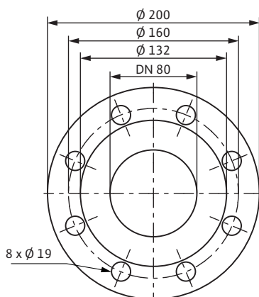
Flange PN 10 for DN 80
