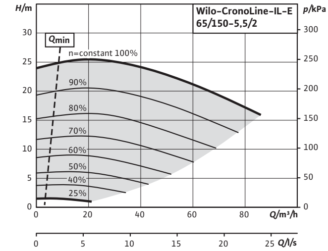
CronoLine-IL-E 65/150-5,5/2 (2 poli)
