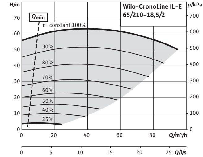
CronoLine-IL-E 65/210-18,5/2 (2 poli)
