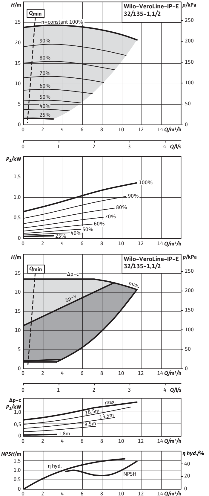
Veroline-IP-E 32/135-1,1/2
