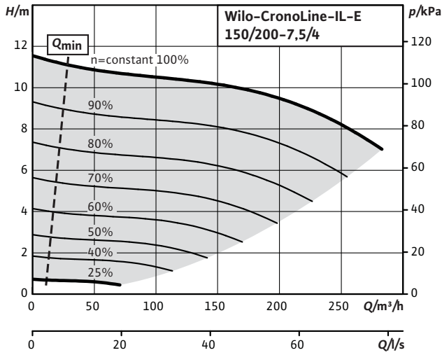
CronoLine-IL-E 150/200-7,5/4 (4 poli)
