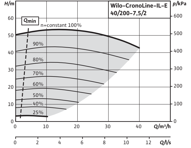
CronoLine-IL-E 40/200-7,5/2 (2 poli)
