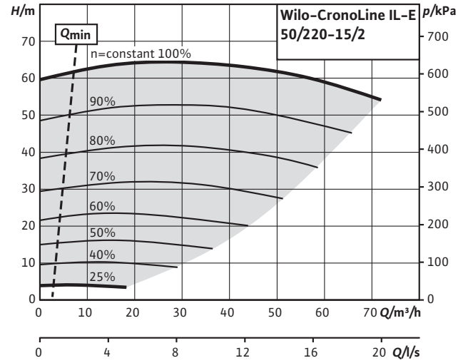
CronoLine-IL-E 50/220-15/2 (2 poli)
