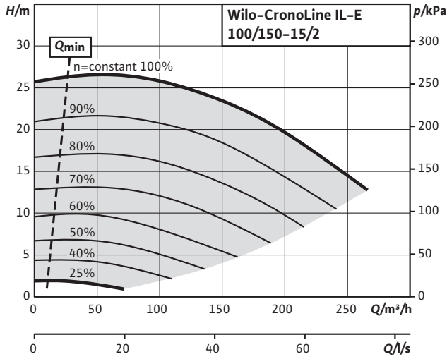
CronoLine-IL-E 100/150-15/2 (2 poli)
