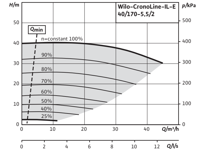
CronoLine-IL-E 40/170-5,5/2 (2 poli)
