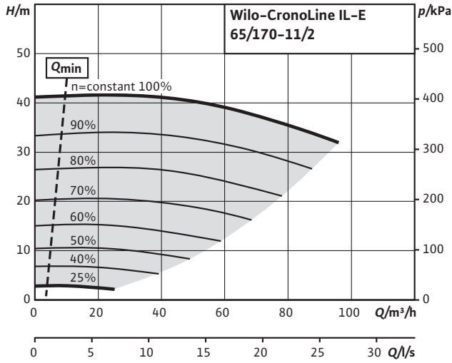
CronoLine-IL-E 65/170-11/2 (2 poli)
