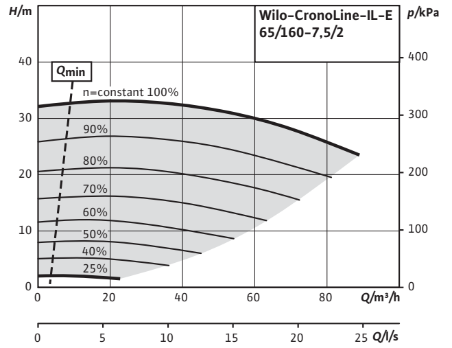
CronoLine-IL-E 65/160-7,5/2 (2 poli)
