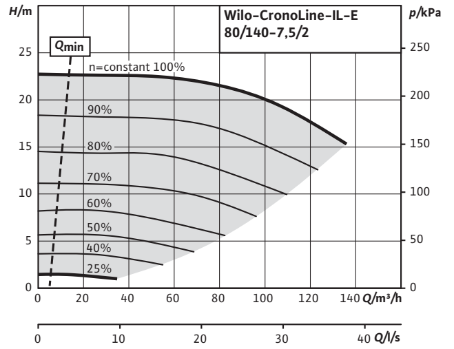
CronoLine-IL-E 80/140-7,5/2 (2 poli)
