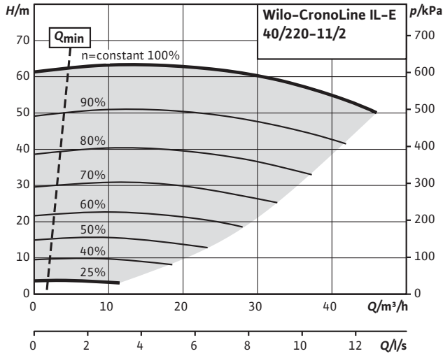
CronoLine-IL-E 40/220-11/2 (2 poli)
