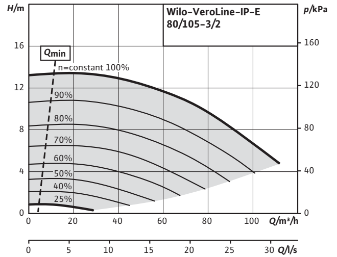
VeroLine-IP-E 80/105-3/2
