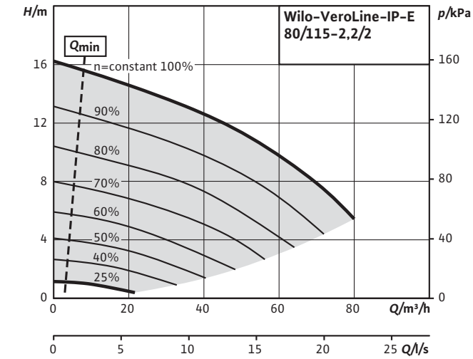
VeroLine-IP-E 80/115-2,2/2
