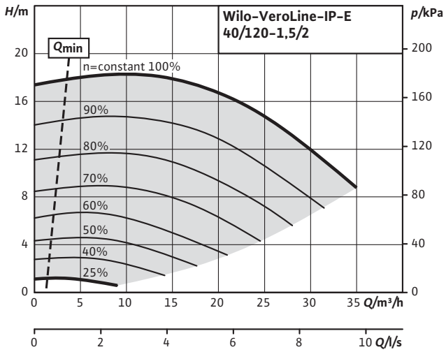
Veroline-IP-E 40/120-1,5/2
