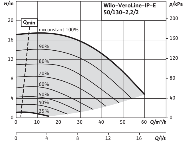
Veroline-IP-E 50/130-2,2/2
