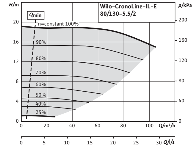
CronoLine-IL-E 80/130-5,5/2 (2 poli)
