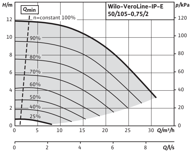
Veroline-IP-E 50/105-0,75/2
