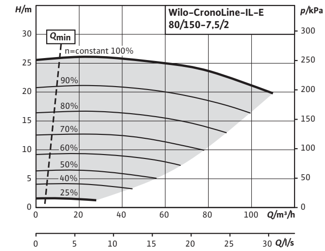
CronoLine-IL-E 80/150-7,5/2 (2 poli)
