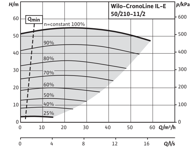
CronoLine-IL-E 50/210-11/2 (2 poli)
