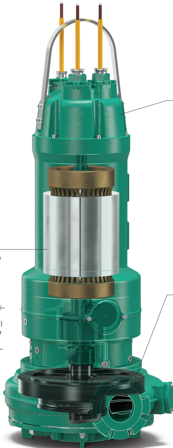
Wilo-EMU FA mit SOLID-G-Lauftrad und FKT-Motorentechnologie
